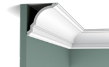
CX106 | CX106F 200 x 11,8 x 11,7 cm Duropolymer®
